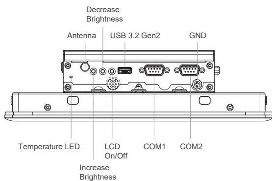
Left I/O
