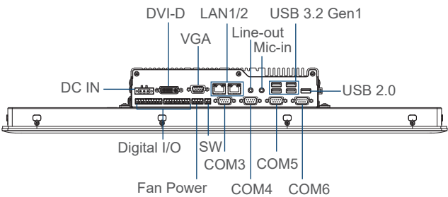
Left I/O
